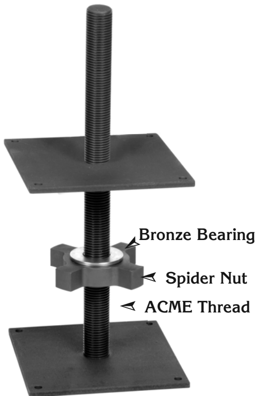
6680 Leveler
